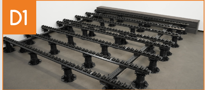
Ersten KL-Kreuzverbinder fixieren und Ausrichtung prüfen
