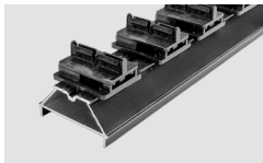
QLICK Alu-UK Alu-Systemschienen (inkl. Befestiger) mit statischer Belastbarkeit
