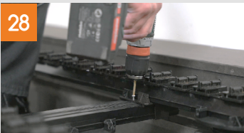
Montage der Terrassendielen in der Fläche
