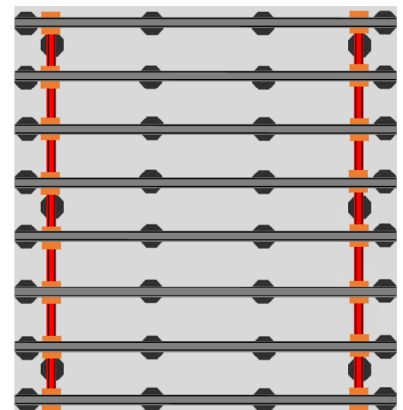
KL-Kreuzverbinder Der KL-Kreuzverbinder fixiert die tragenden QCLICK Alu-UK mit der TWIXT-Isostep als Konterlatte
